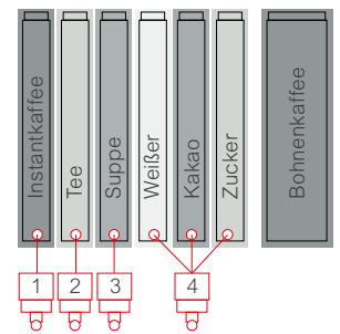
Variante 6405 1 großer Bohnenbehälter 6 Produktbehälter, 4 Mixereinheiten
